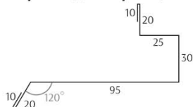
Ветровая доска фальцевая
