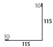
Уголок наружный 115*115
