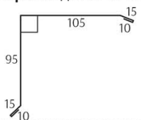
Ветровая доска 95*120
