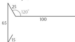
Торцевая планка
