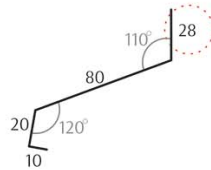
Планка отлива 80 под заглушку
