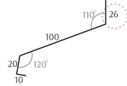
Планка отлива 100 под заглушку
