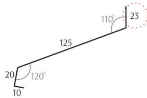
Планка отлива 125 под заглушку
