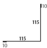
Уголок внутренний 115*115
