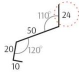
Планка отлива 125 под заглушку
