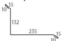
Планка примыкания верхняя
