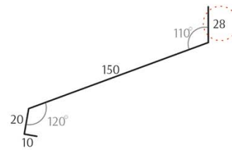
Планка отлива 150 под заглушку
