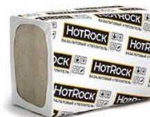
Утеплитель базальтовый ХотРок Вент Про 75 кг/м 3 1200*600*100 (2,16м 2 0.216м 3 )
