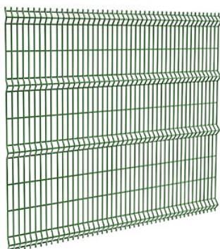
Секция сварная 3D/Гиттер 1530*2500 4мм (яч.50x200)
