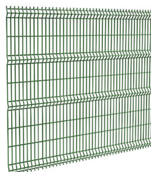
Секция сварная 3D/Гиттер 1530*2500 3мм (яч.50x200)
