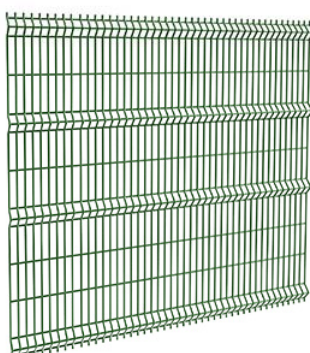
Секция сварная 3D/Гиттер 1500*2500 5мм (яч.50x200)
